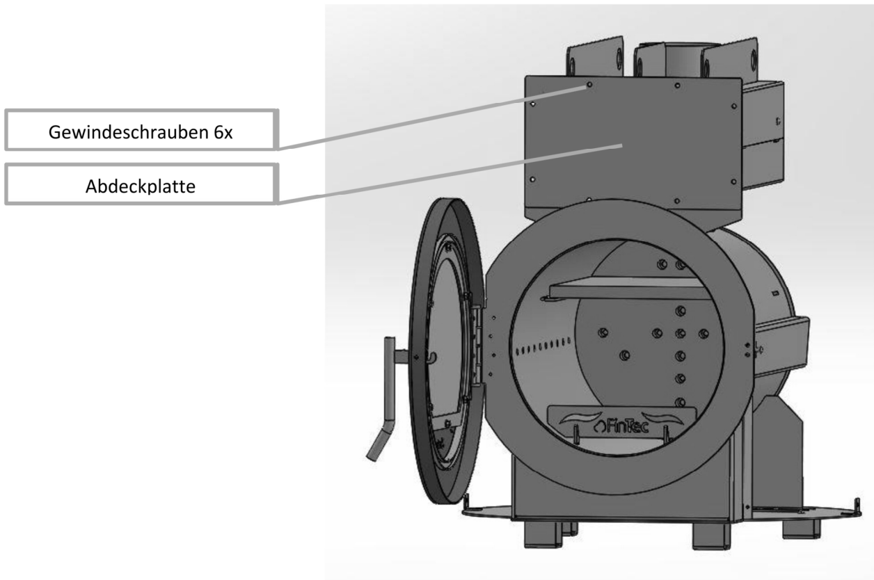
Abbildung 3: Reinigung Nachbrennkasten
