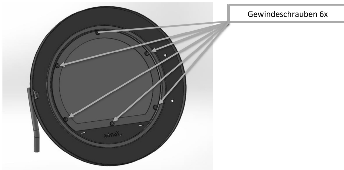
Abbildung 2: Fixierung Glasscheibe
