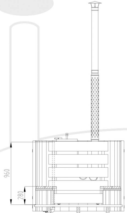
SCHNITT A-A
