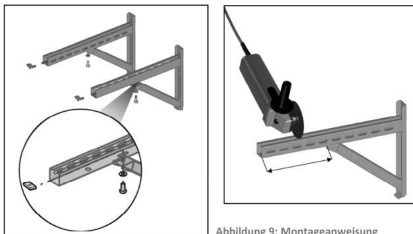
Abbildung 9: Montageanweisung Querträger
