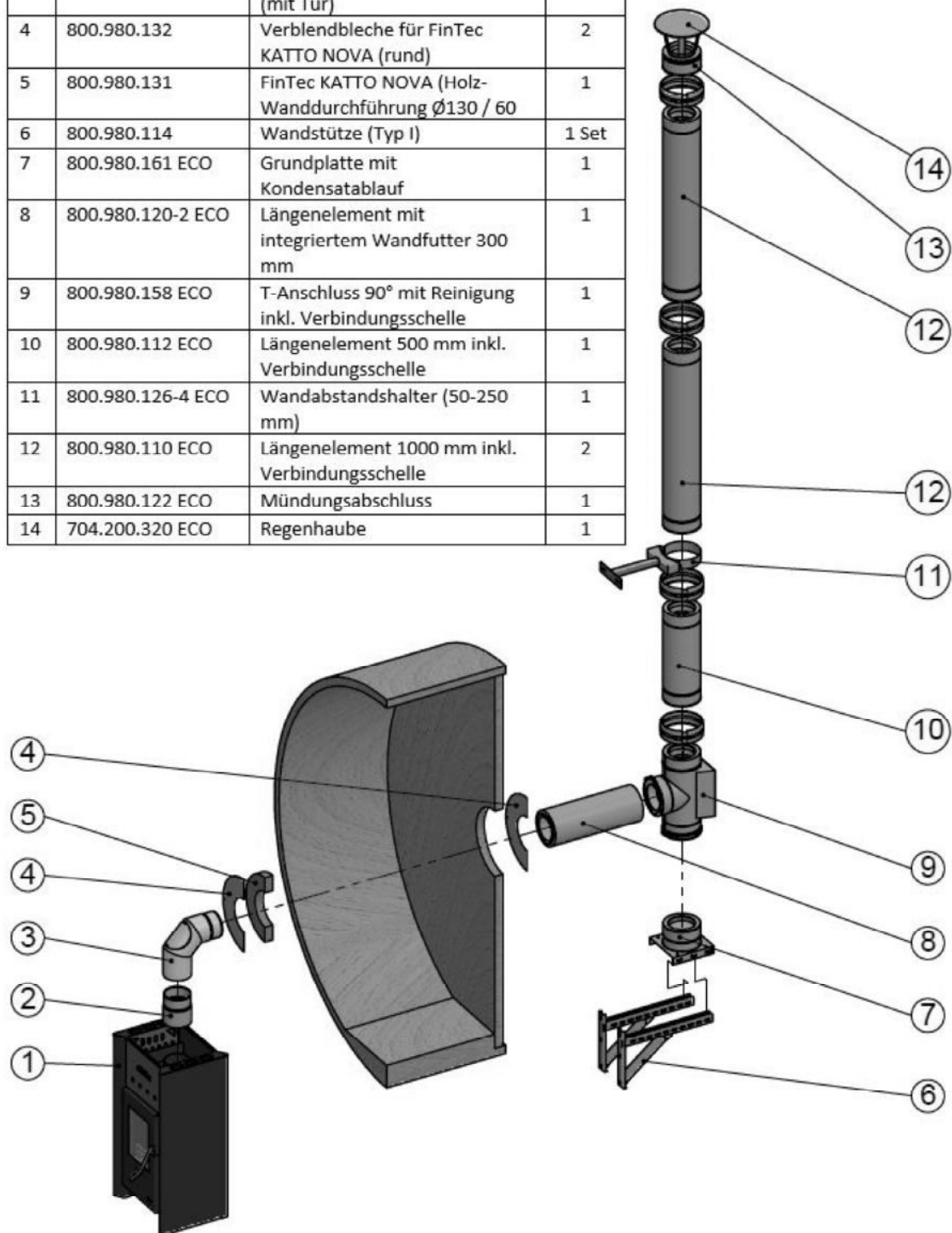
Abbildung 1: Lieferumfang
