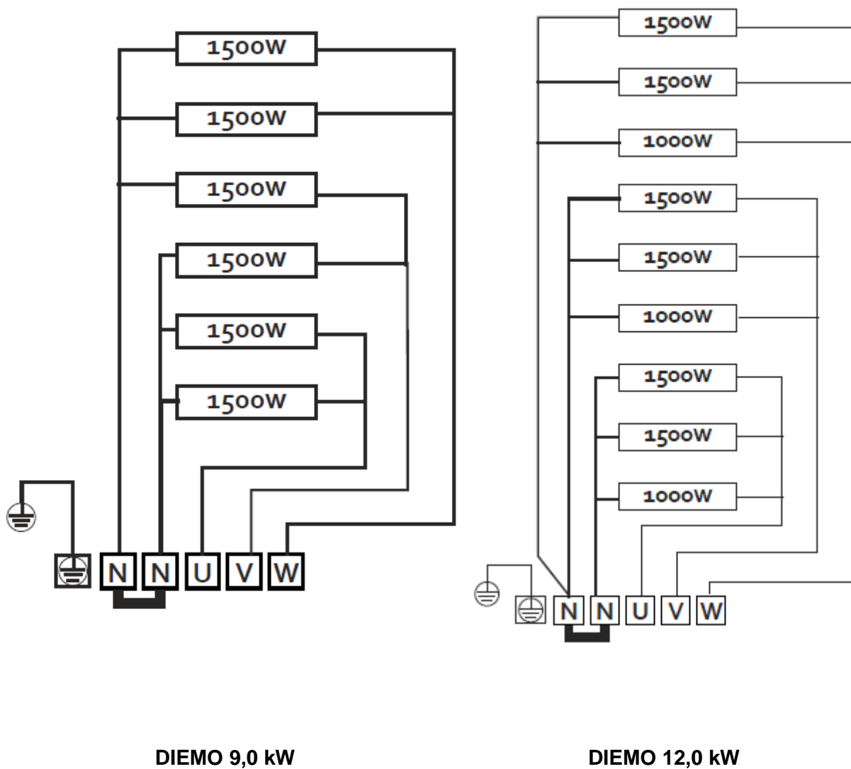
Abbildung 1: Anschlussplan
